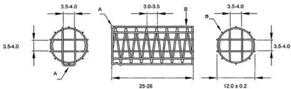
Рисунок 2.1.9.3.-3. – Альтернативное приспособление для погружения (размеры в миллиметрах). А – кислотоустойчивый проволочный зажим; В – кислотоустойчивая проволочная основа.
